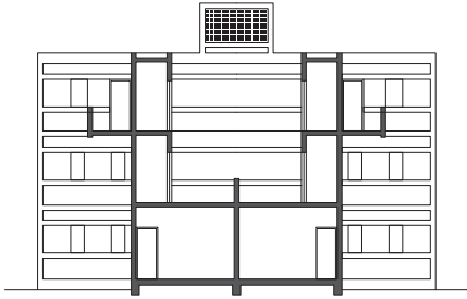
Section D2/E2
